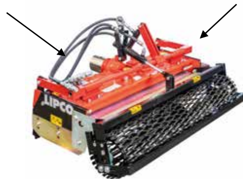
Hydraulische Tiefenregulierung über die Walze und hydr. Einstellung des Standard-Planierschildes
